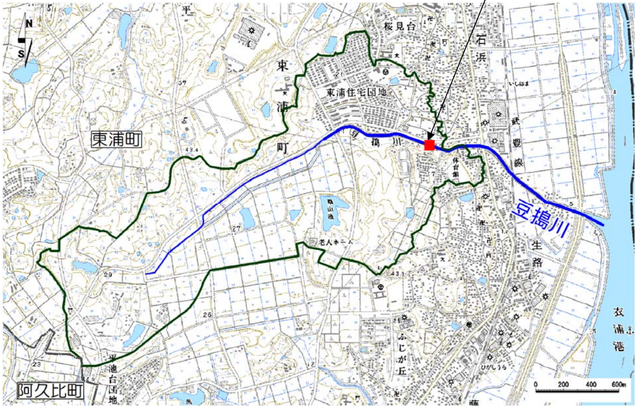
(参考図) 豆搗川水系図
