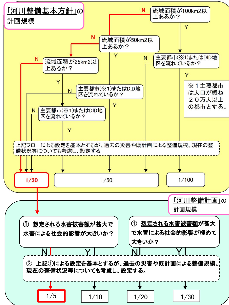
▲ 計画規模決定フロー
