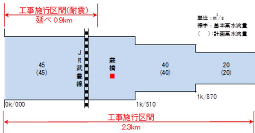
図 3.1.2 河川整備計画の目標とする流量配分図(m³/s)
