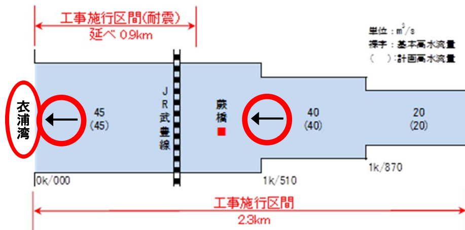
図 3.1.2 河川整備計画の目標とする流量配分図(m³/s)
